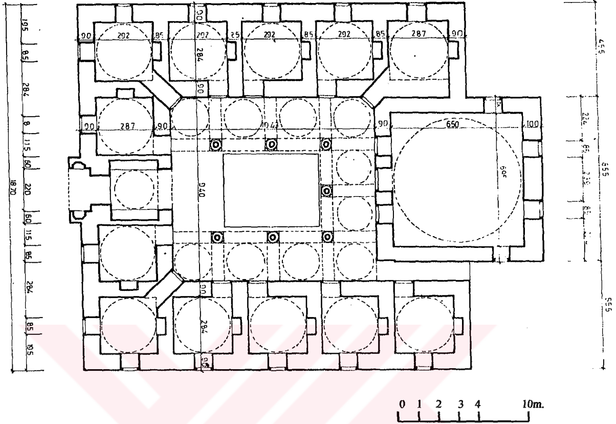
Şekil II: Gazi Hüsrev Bey Medresesinin bir plan örneği
