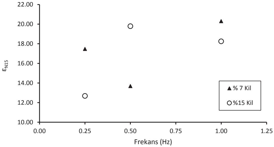
Şekil 4.9. Frekansa karşılık 15. çevrimdeki aksenal deformasyon
