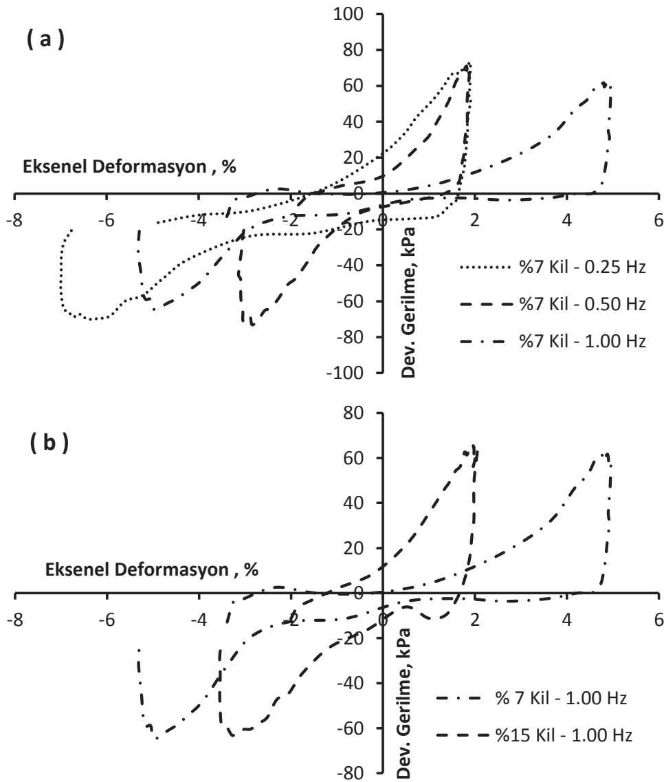
Şekil 4.19. Çevrimdeki ( N_3 ) Eksenel deformasyon (%) – Deviyatör gerilme ( \sigma_d , kPa) ilmikleri.
