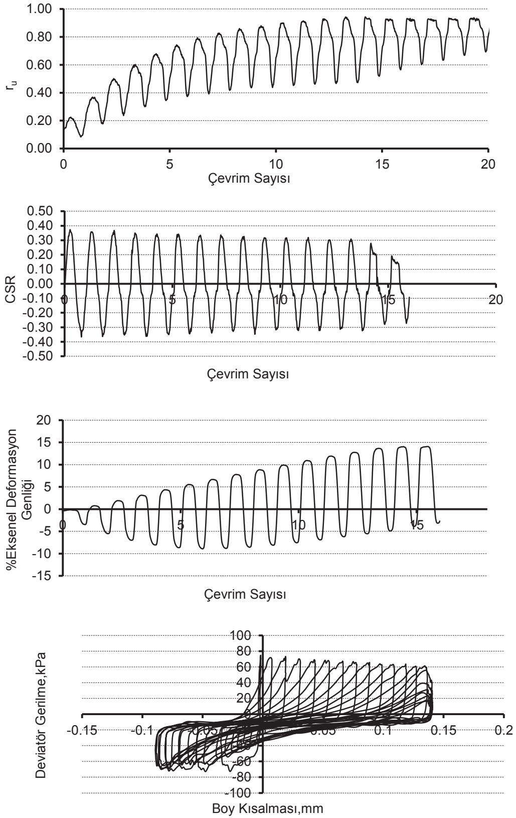
Şekil 4.1. %7 Kil 0.25 Hz deney grafikleri
