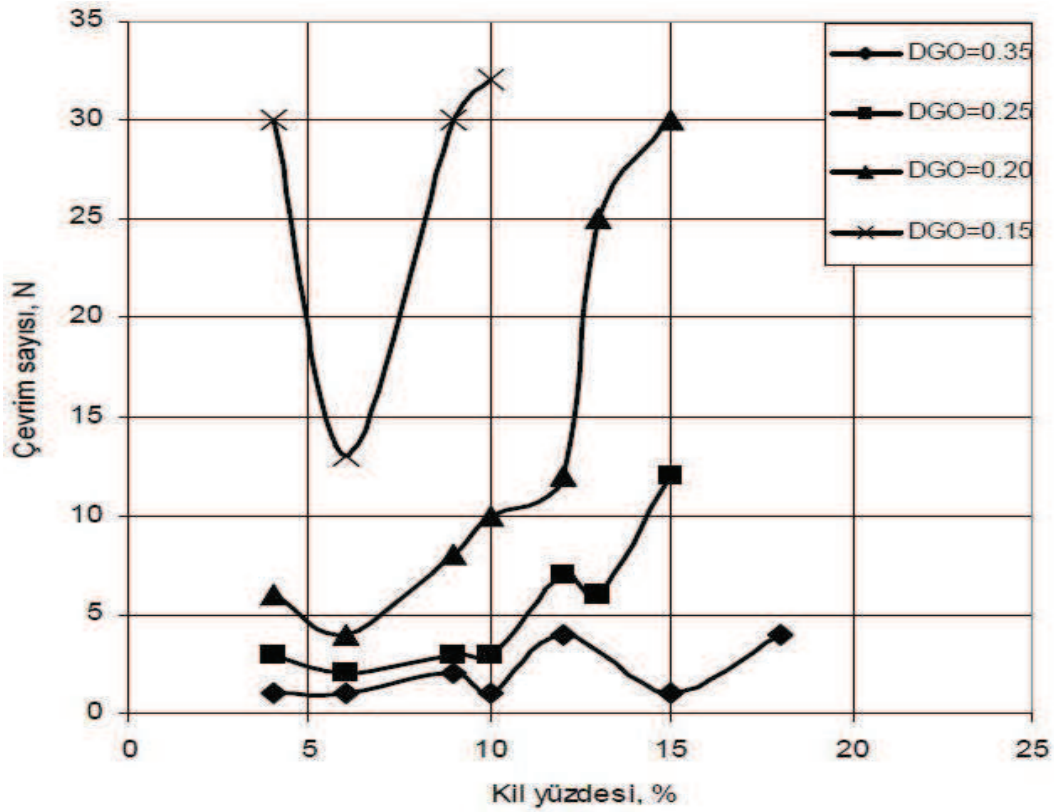
Şekil 2.3. Farklı kil içerikli numunelerde, \pm\%2,5 aksel deformasyon seviyesine ulaşması için gerekli çevrim sayısı – kil yüzdesi bağıntısı [1]
