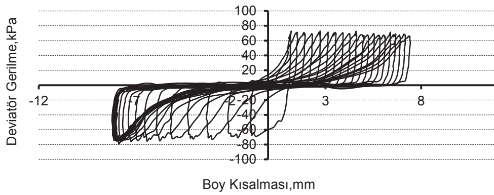
Şekil 4.2. %7 Kil 0.50 Hz deney grafikleri
