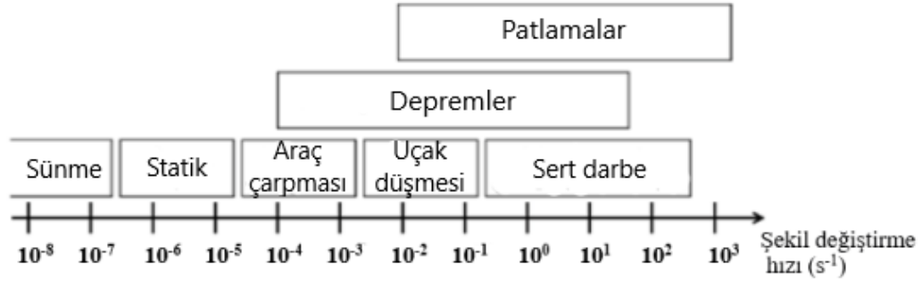
Şekil 2.5. Farklı yüklemeye türlerinde şekil değiştirme hızları (Hentz ve ark., 2004)
