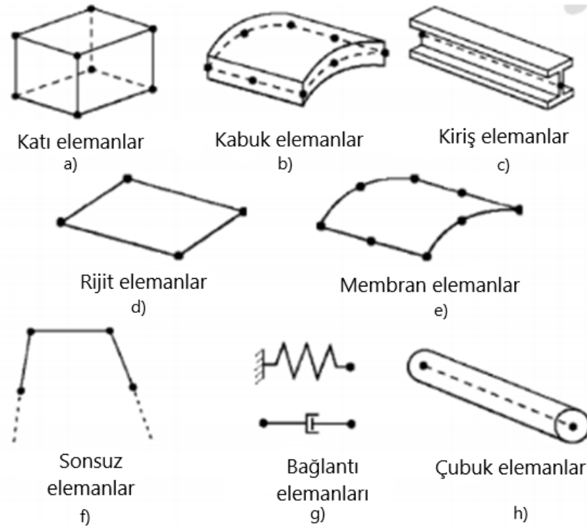
Şekil 3.6. Eleman türleri
