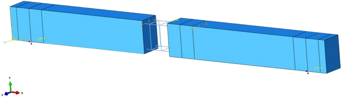
Şekil 4.22. UH-S13 numunesi sonlu eleman modeli
