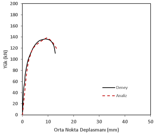
Şekil 4.28. UH-N numunesi Yük-Deplasman grafiği
