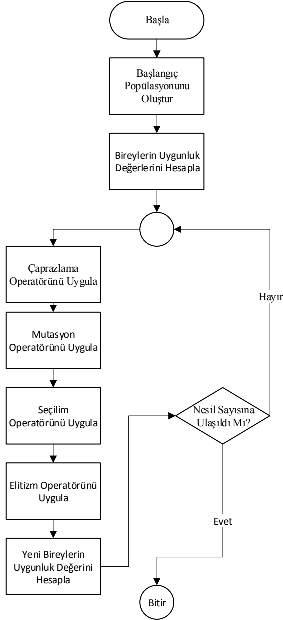
Şekil 5.6. Genetik algoritma akış diyagramı
