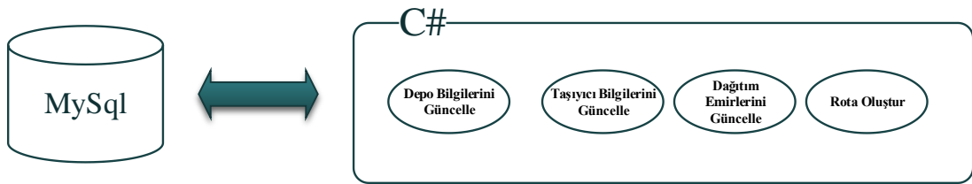
Şekil 5.1. Nesnelere arası program akışı
