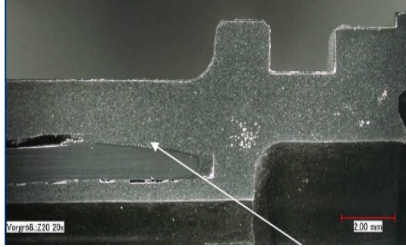
Şekil 4.10. PA12LX9013 Kaynak bölgesi
