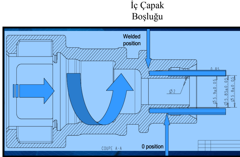
Şekil 3.26. Kopmenant ile borunun kaynak bölgesi resmi
