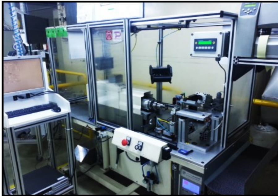
Şekil 3.6. Spinwelding makinası
