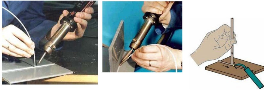
Şekil 1.1. Sıcak gaz kaynağı (1)
