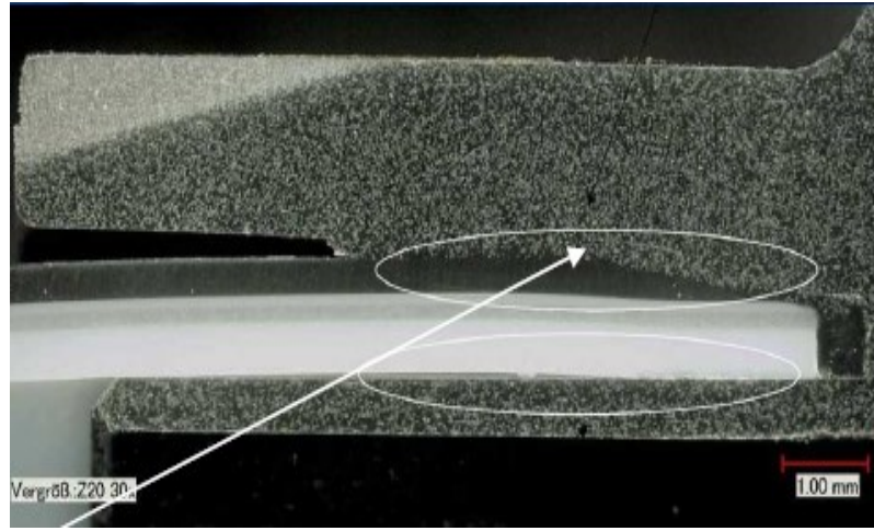
Şekil 4.11. MLT 4300 Kaynak bölgesi
