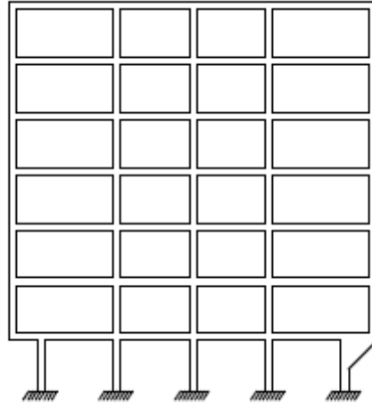
Şekil 3.4. Kolonların konsol ve guselere oturtulması
