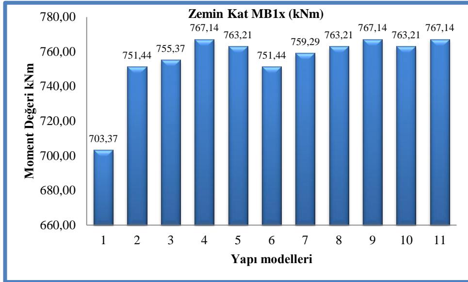
řekil 5.42. B1 Kolonunun yapı modellerine göre zemin kat x doęrultusunda moment deęiřimi
