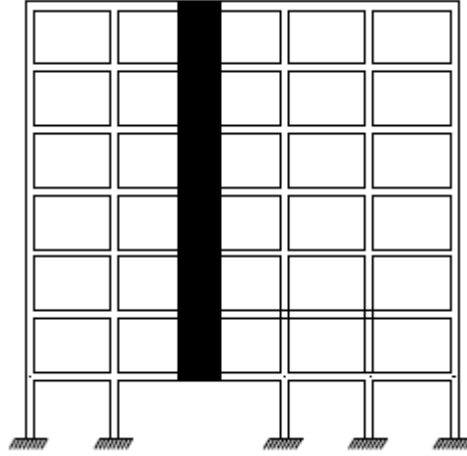
Şekil 3.7. Perdenin kirişe oturması durumu
