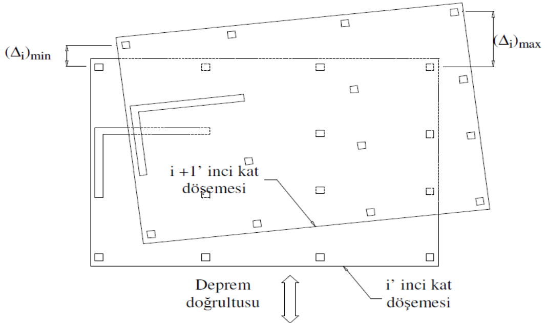
Şekil 3.1. Burulma düzensizliği
