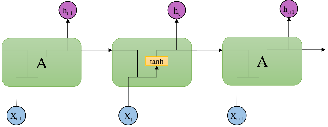
Şekil 3.4: Standart RNN'deki Yinelenen Tek Katman
