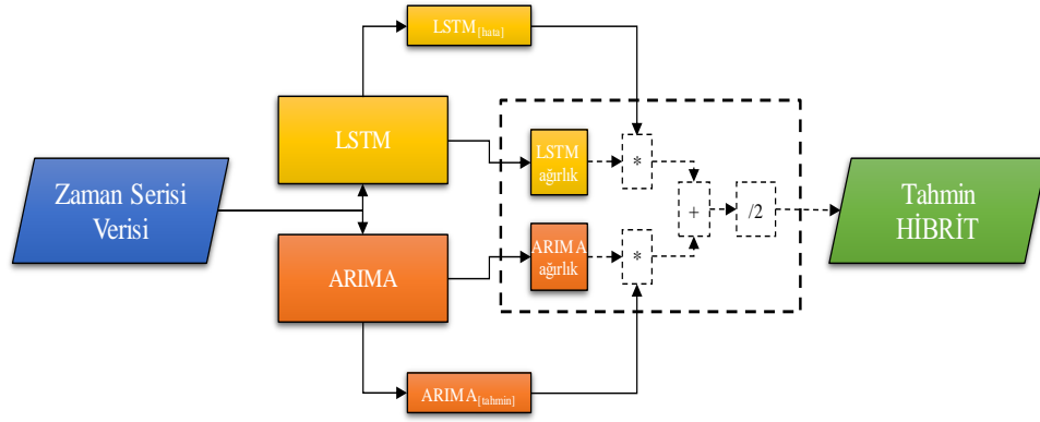
Şekil 3.19: Hibrit Model Diyagramı
