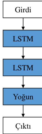
Şekil 3.15: Yığılmış LSTM Mimarisi
