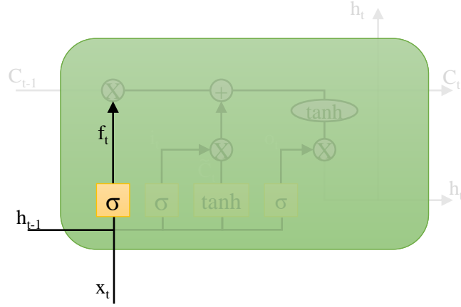
Şekil 3.11: LSTM İçindeki Unutmaya Kapısının Gösterimi
