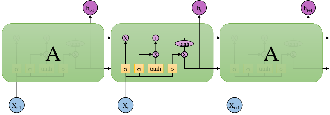
Şekil 3.6: LSTM'deki Etkileşimli Dört Katman
