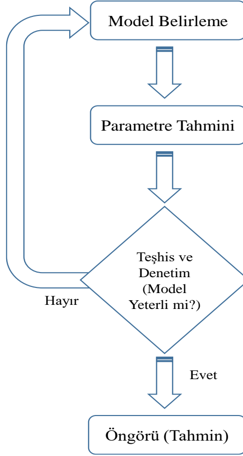
Şekil 3.1: ARIMA Modelinin Akış Şeması
