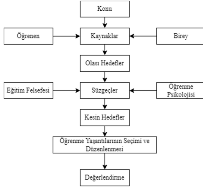
Şekil 2: Tyler Modeli
