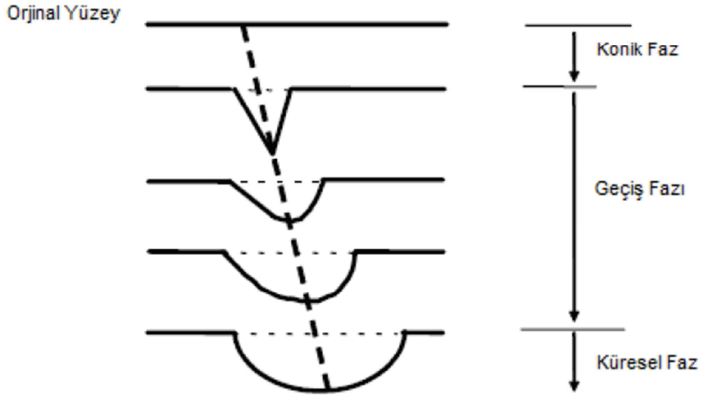
Şekil 2.7. İzlerin banyo süreci boyunca aldığı şekiller.
