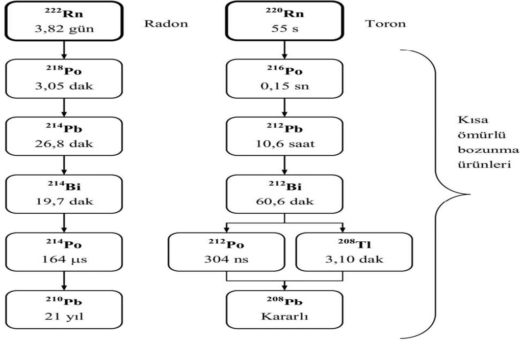
Şekil 2.2. Radon gazının (Rn-222) bozunum ürünleri ve bozunum süreleri
