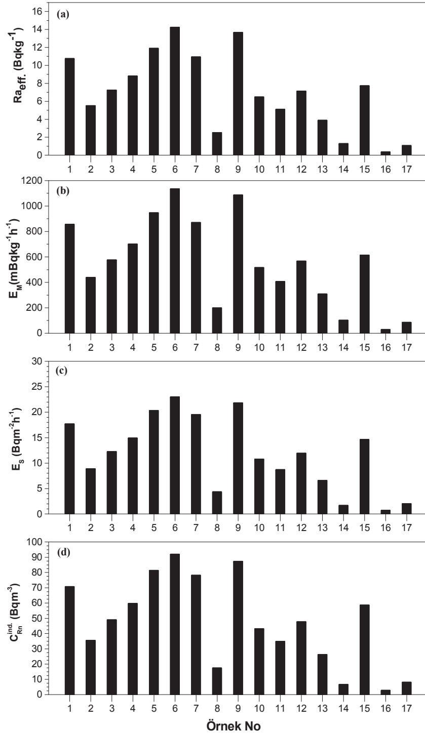
Şekil 3.4. Orhaneli (1-14) ve DOSAB (15-17) bölgesindeki topraklarda efektif radyum içeriği (a), kütle eksalasyon oranları (b), yüzey eksalasyon oranları (c) ve iç mekan radon aktivitesine katkıları (d).
