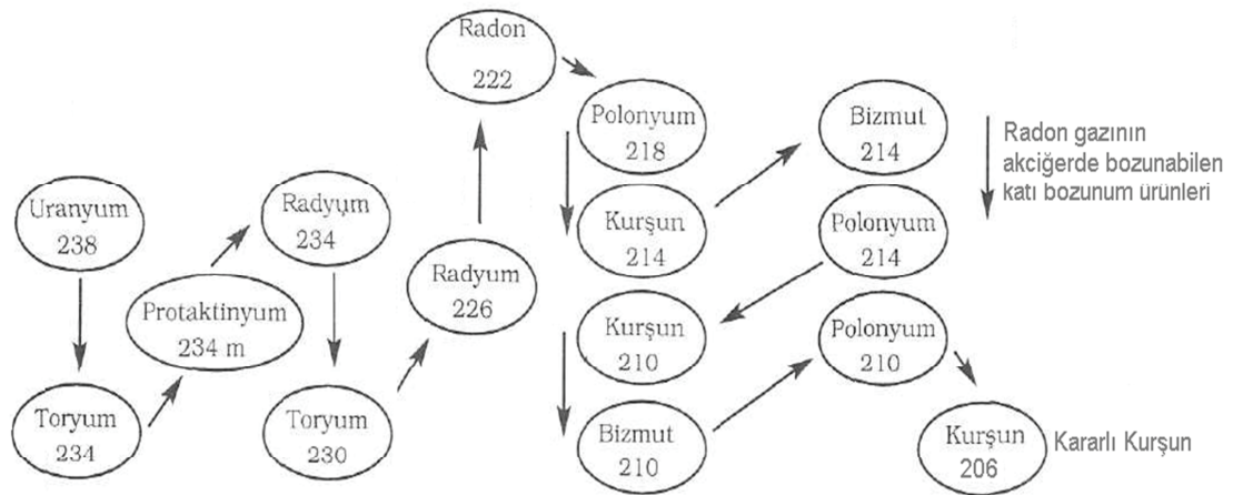
Şekil 1.1. Uranyum serisi ve radonun bozunum ürünleri
