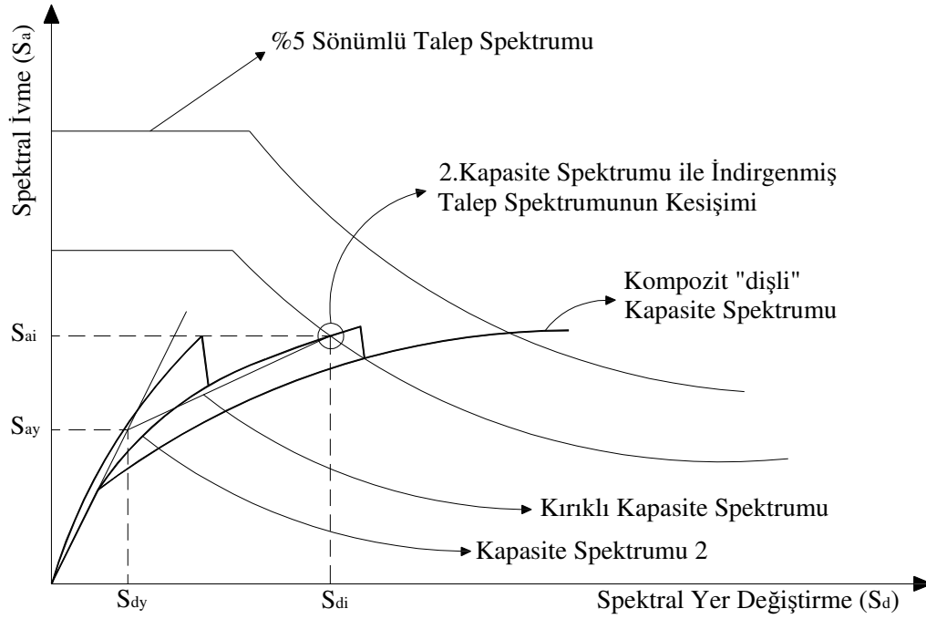
Şekil 3.12. Talep ve kompozit (dişli) kapasite spektrumlarının kesişim noktası [2]
