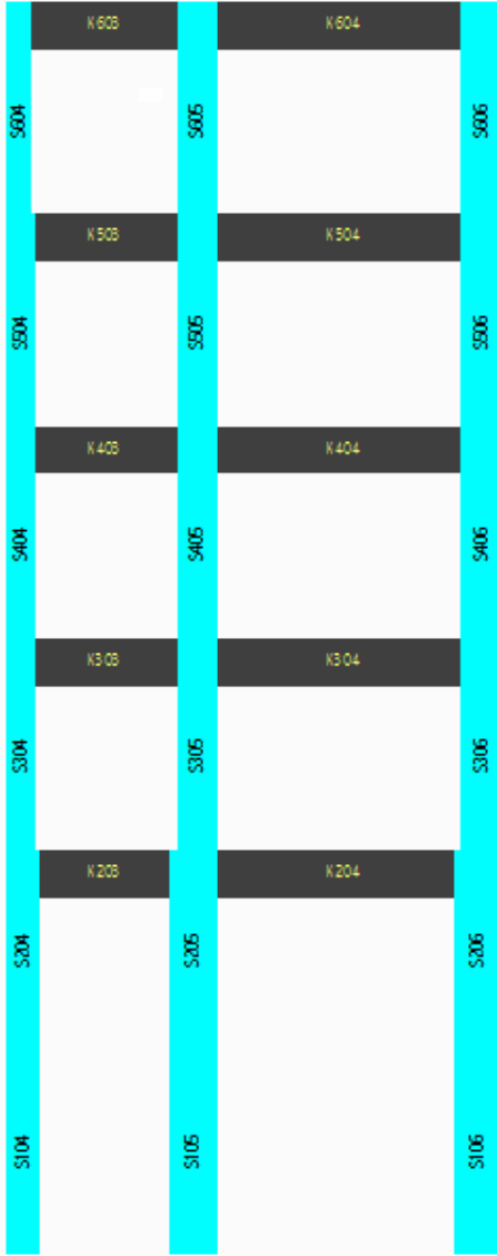
Şekil 4.3. Mevcut yapıya ait X doğrultusunda, E aksı boy kesiti
