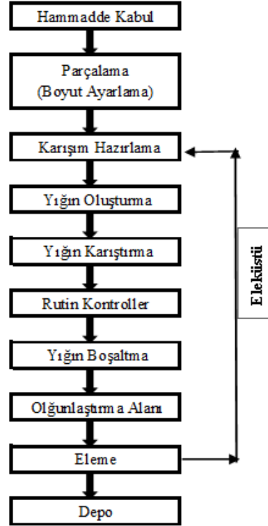
Şekil 2.7. Windrow Kompost Yöntemi İş Akım Şeması
