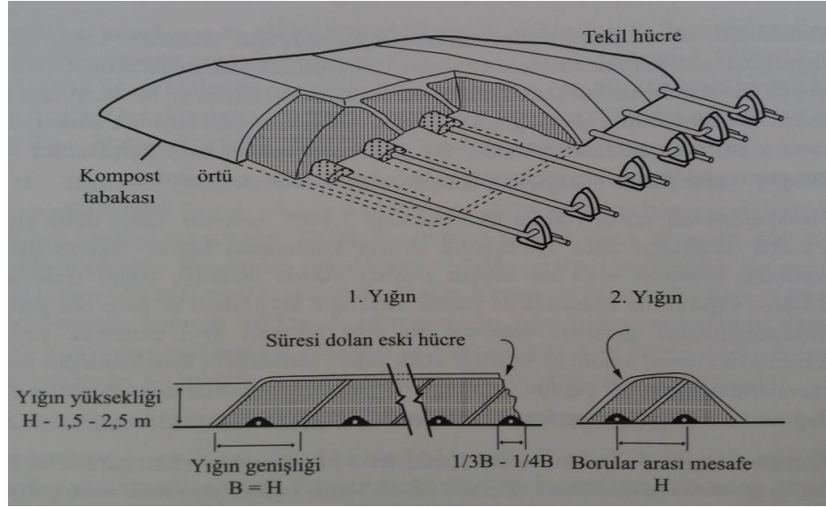
Şekil 1.7. Hücre Eklemeli Havalandırılmalı Statik Yığın [7]
