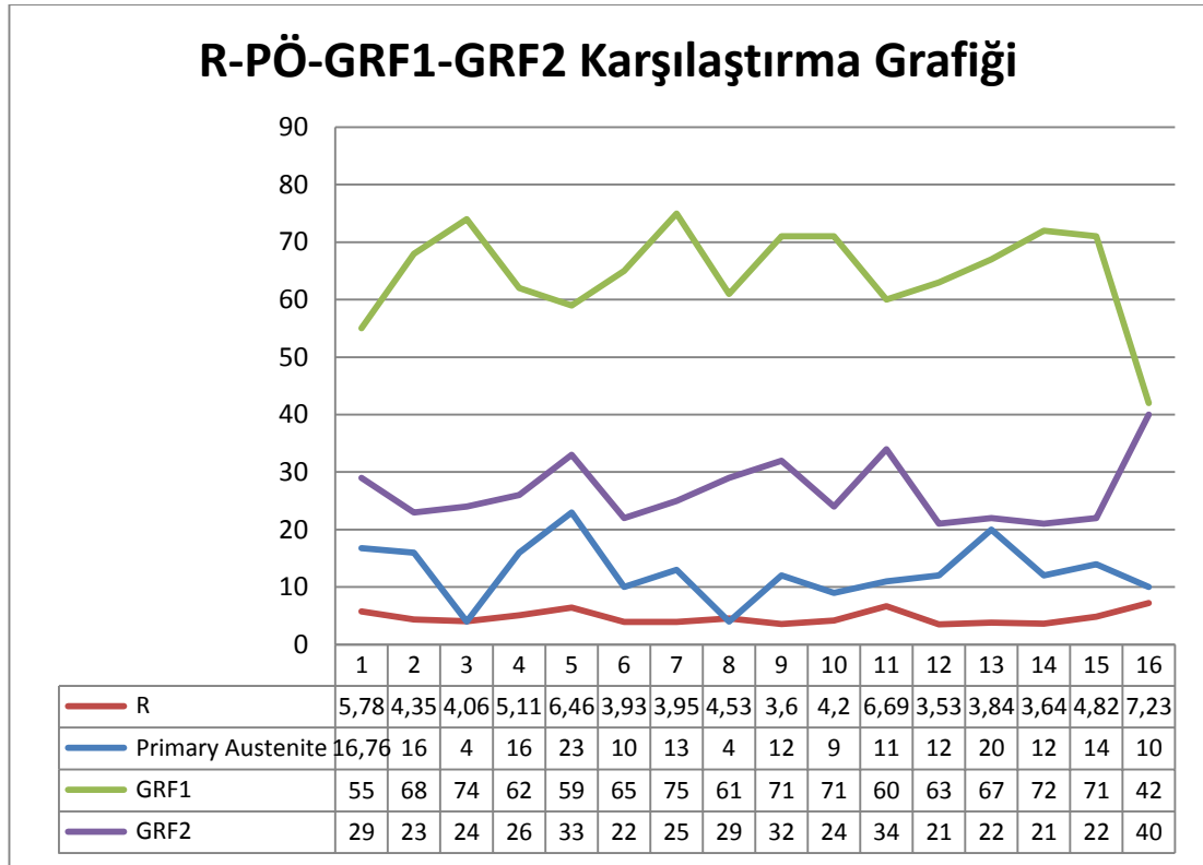
Şekil 5.35. R-PÖ-GRF1-GRF2 Karşılaştırma grafiği
