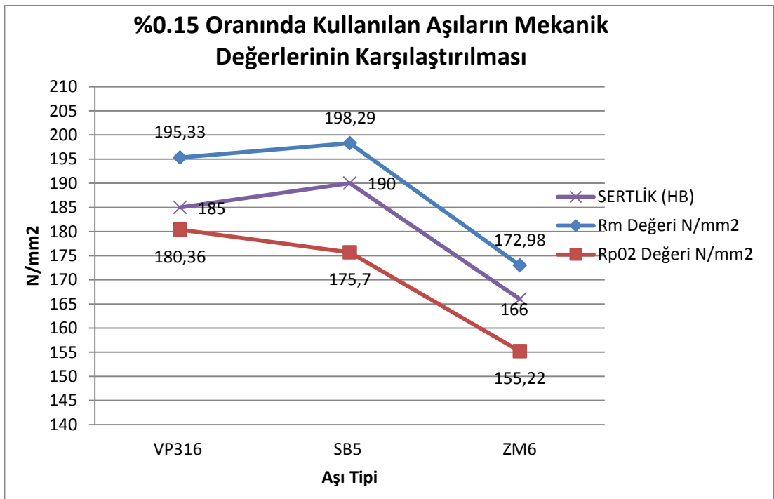
Şekil 5.29. GG25 Malzeme için ; farklı aşu tiplerinin %0.15 oranında kullanılmasının mekanik değerlere etkisinin grafiği
