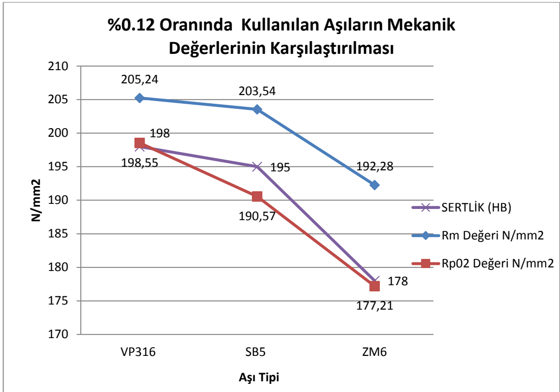
Şekil 5.28. GG25 Malzeme için ; farklı aşu tiplerinin %0.12 oranında kullanılmasının mekanik değerlere etkisinin grafiği
