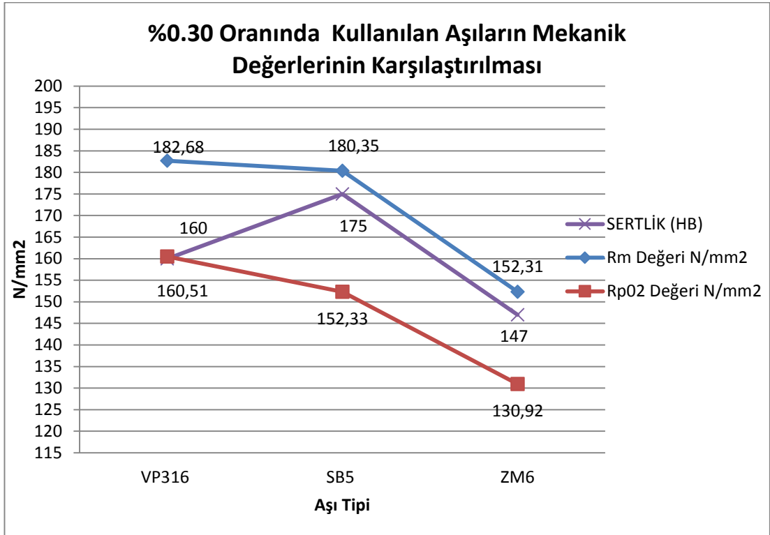
Şekil 5.32. GG25 Malzeme için ; farklı aşılarda kullanılması mekanik değerlere etkisinin grafiği
