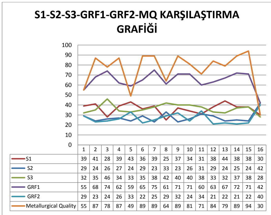
Şekil 5.36. S1-S2-S3-GRF1-GRF2-MQ Karşılaştırma grafiği
