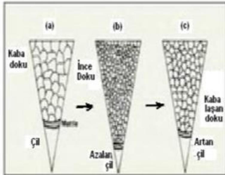
Şekil 1.1. Aşılamanın kama numunelerinde görülen ötektik hücre sayısı ve chill derinliğine etkisi, (a) Aşılama öncesi, (b) Aşılama sonrası, (c) Aşılama sonrası döküme kadar uzun süre geçmesi nedeniyle aşılama sonumu
