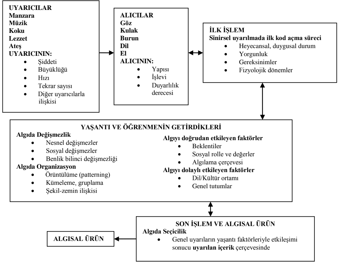
Şekil 2. Algılama Modeli
