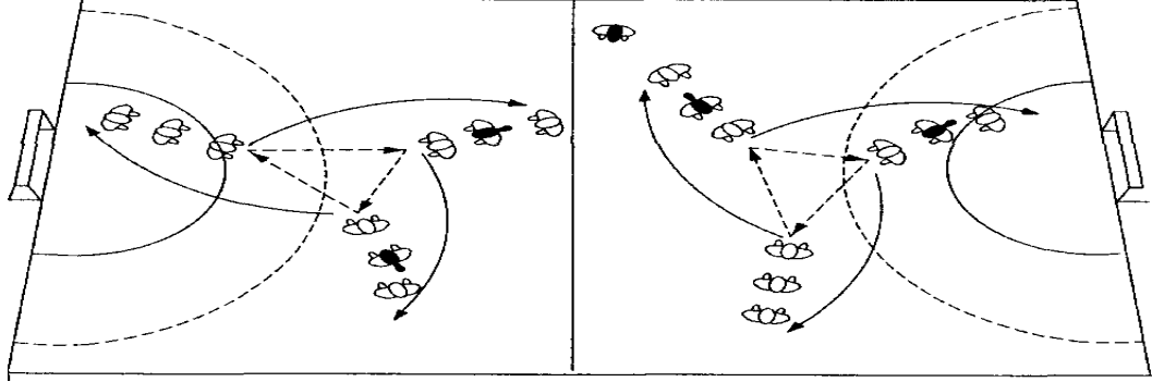
Şekil 2. Üçgende paslaşma
